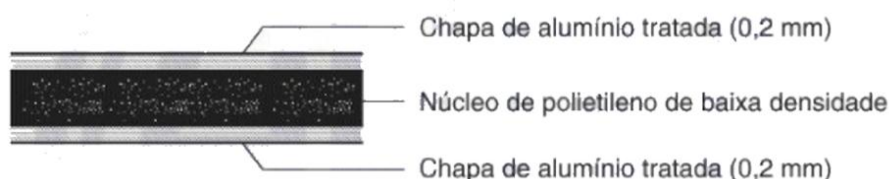
Figura 1: Chapa de alumínio composto - Material e espessura
